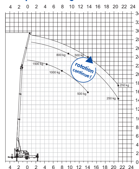
Abaque de charge
