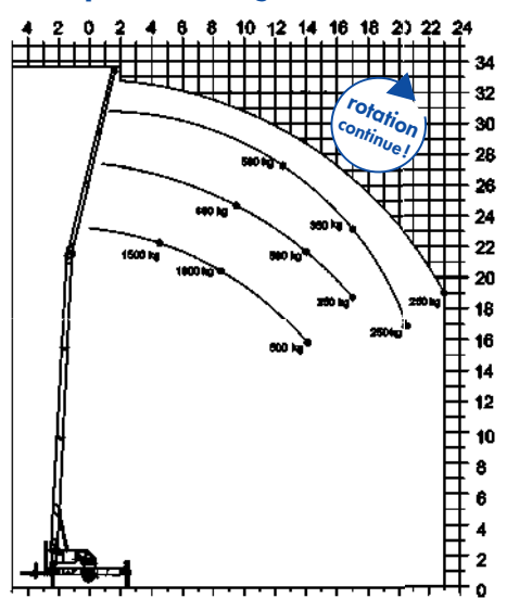
Abaque de charge
