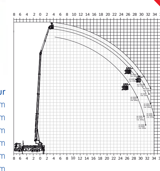
Abaque de nacelle
