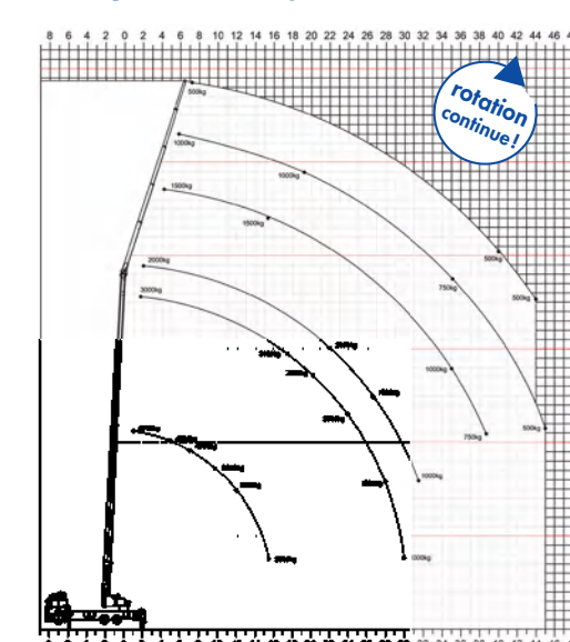
Abaque de charge
