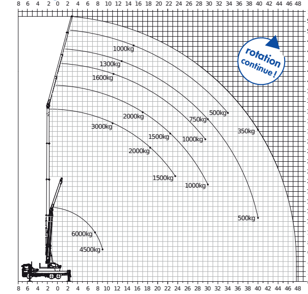
Abaque de charge
