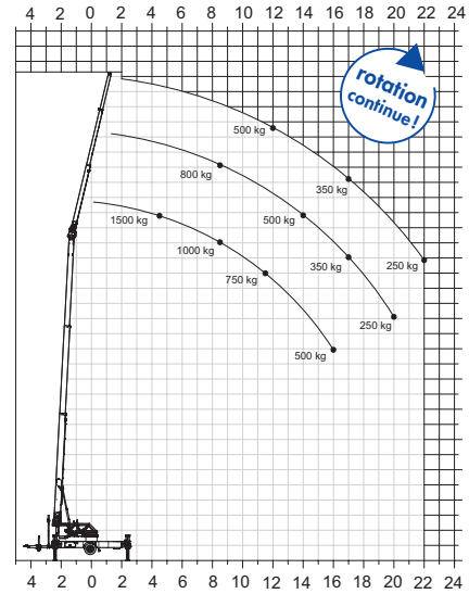
Abaque de charge
