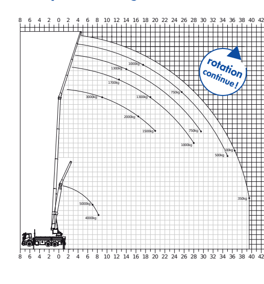
Abaque de charge
